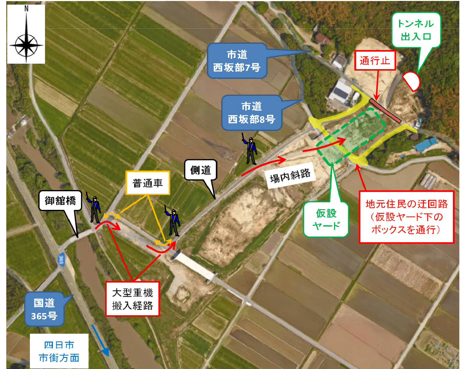
【大型重機の搬入ルート図】
