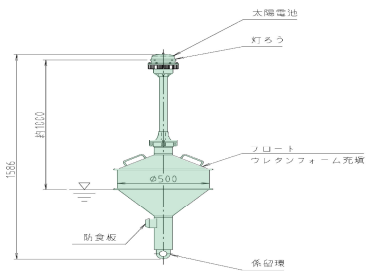
灯浮標参考図
