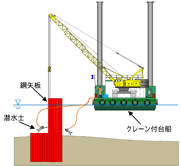
鋼矢板切断状況図
