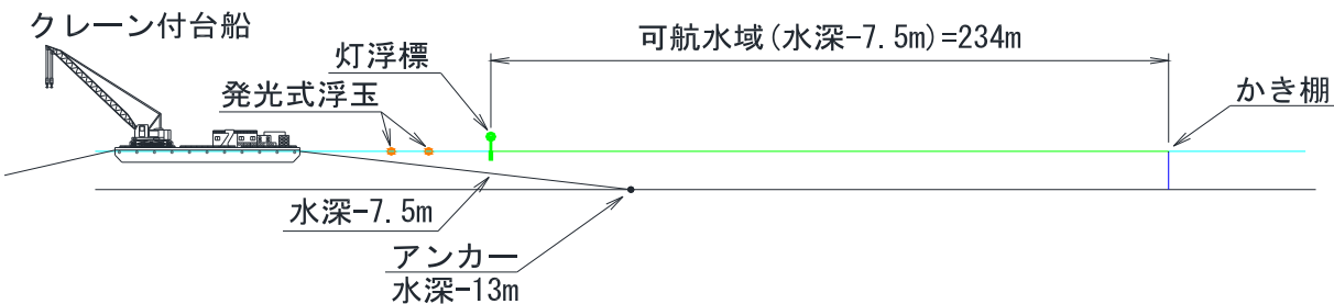
作業区域航路断面図
