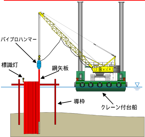
鋼矢板打設状況図
