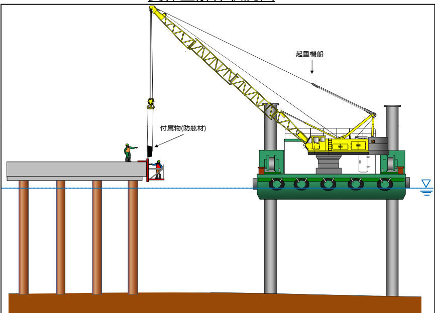
付属物設置状況図
