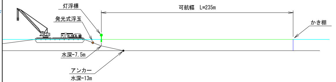
作業区域航路断面図
