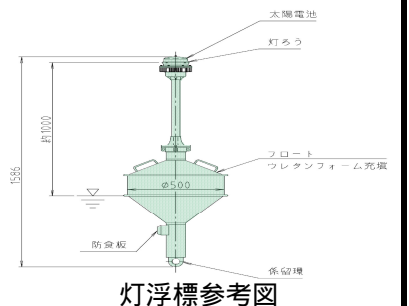
灯浮標参考図
