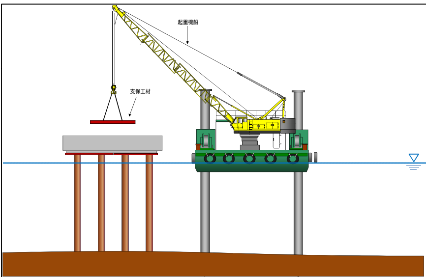
支保工解体状況図
