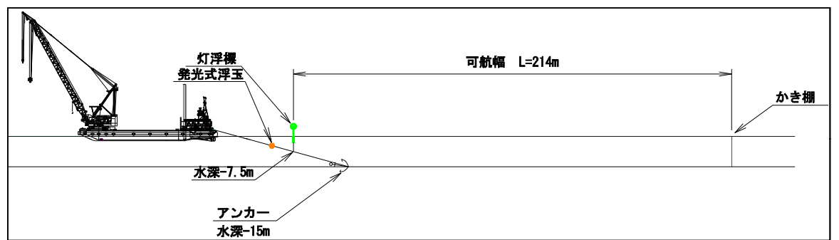
作業区域航路断面図(ホイス・プラットフォーム設置時)
