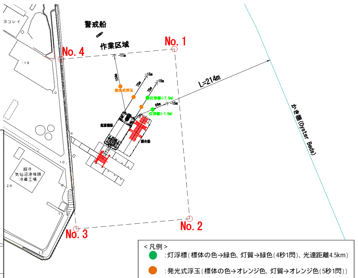
作業区域図(ホイス・プラットフォーム設置時)
