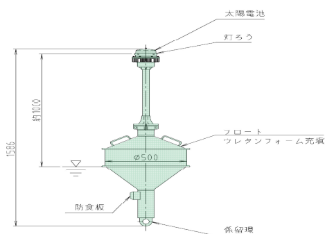
灯浮標参考図
