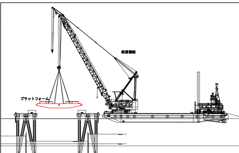
プラットフォーム据付状況図
